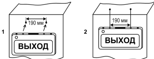
Рис.1 Установка оповещателя
